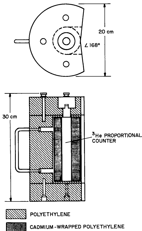
Fig. 22. ^3\text{He} neutron detector.
